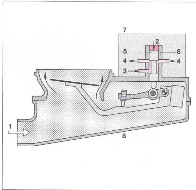
Fig. 15 Cylindre à fentes d'étranglement. 1 Admission d'air 2 Pression de commande 3 Arrivée de carburant 4 Quantité de carburant dosée 5 Piston de commande 6 Cylindre à fentes 7 Doseur-distributeur de carburant 8 Débitmètre d'air
