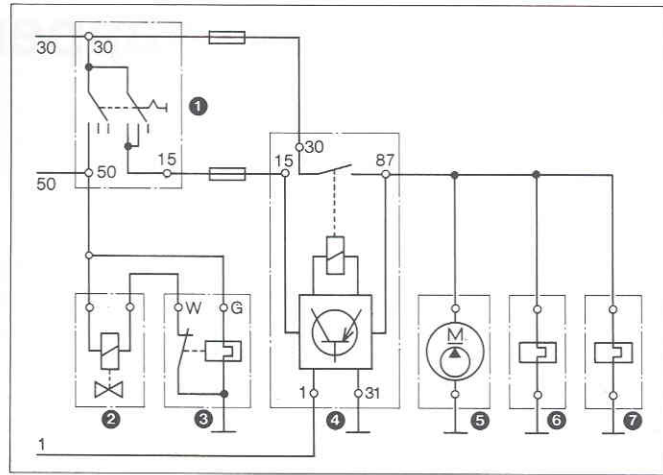
Fig. 38 Circuit en position de repos. 1 Commutateur d'allumage-démarrage 2 Injecteur de départ à froid 3 Thermocontact temporisé 4 Relais de commande 5 Pompe électrique à carburant 6 Correcteur de réchauffage 7 Commande d'air additionnel
